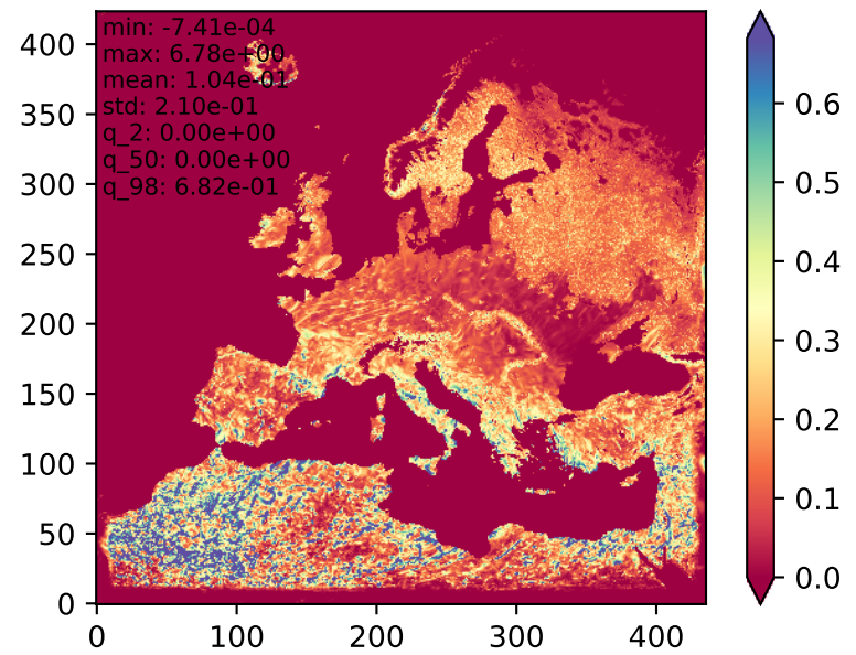
et mean - distribution
